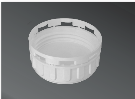
Tapa para Bidón DIN 63 con Oblea Expandida
